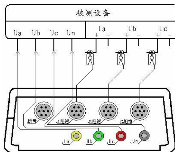
三相四线制设备测试接线图
