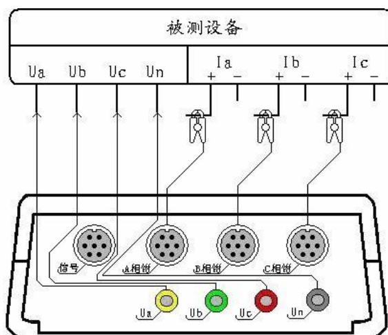
不平衡度测试接线图
