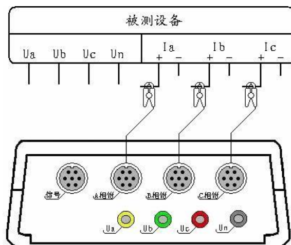
电流谐波测试接线图
